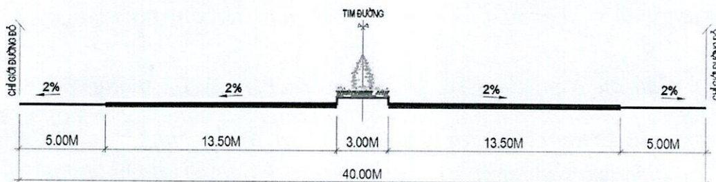
Mặt cắt ngang điển hình đường dẫn
